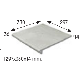
Peldaño recto 60 · Antideslizante Straight stair-tread 60 · Anti slip
