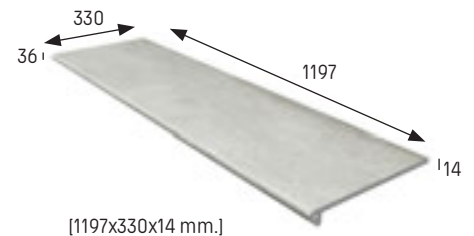
Peldaño recto 120 · Liso Straight stair-tread 120 · Smooth
