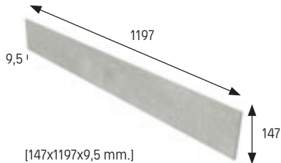
Peldaño recto 30 · Antideslizante Straight stair-tread 30 · Anti slip
